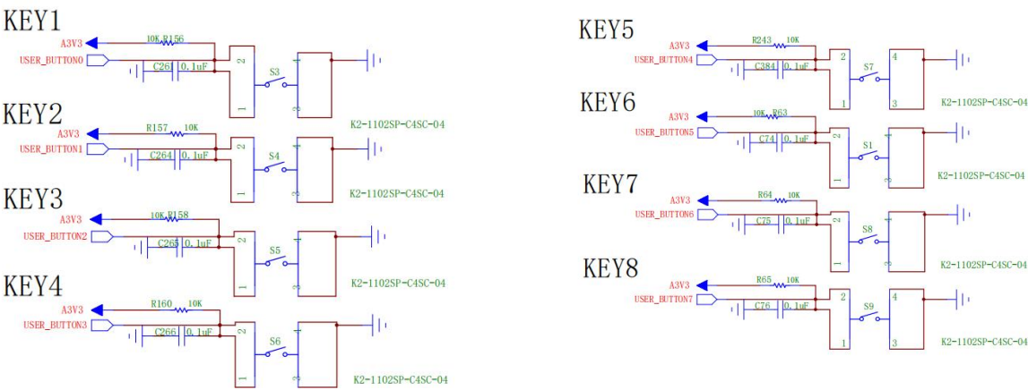
图 3-6 用户按键电路图
