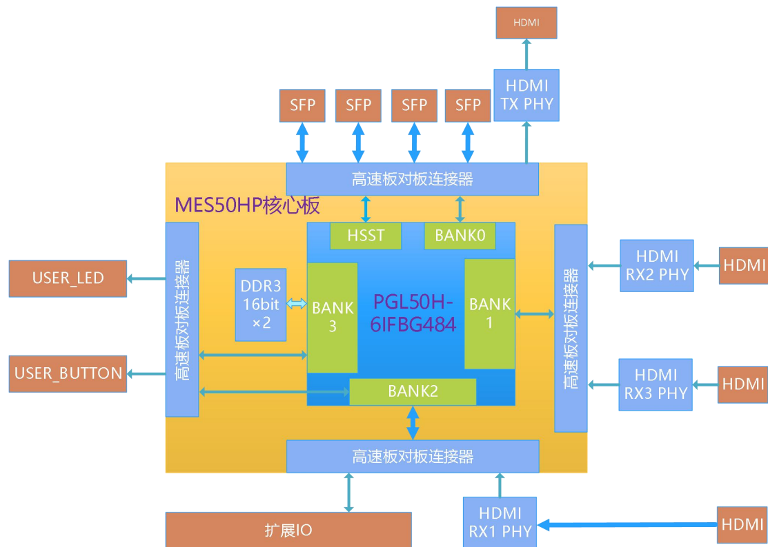
图 1-1 开发系统功能框图
