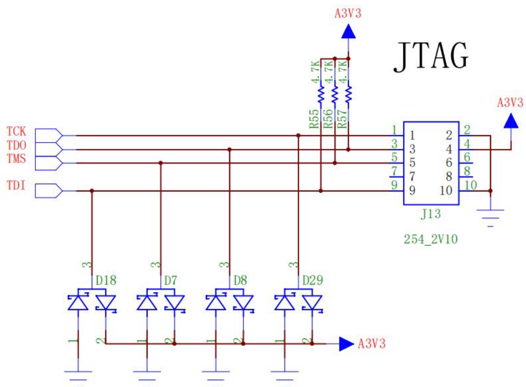
图 3-3 PGL50H JTAG 功能连接图
