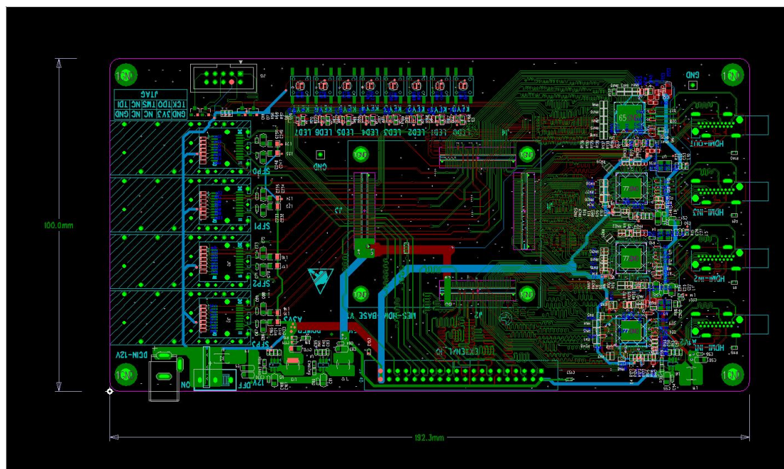
图 3-11 扩展底板尺寸结构图
