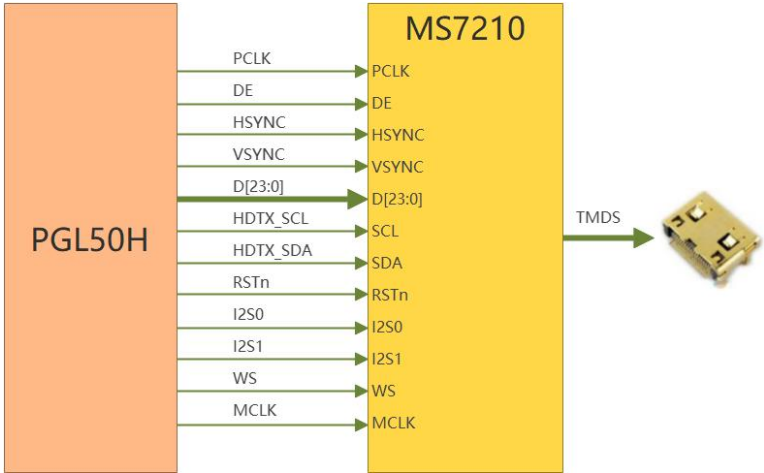
图 3-5 HDMI Transmit 连接示意图
