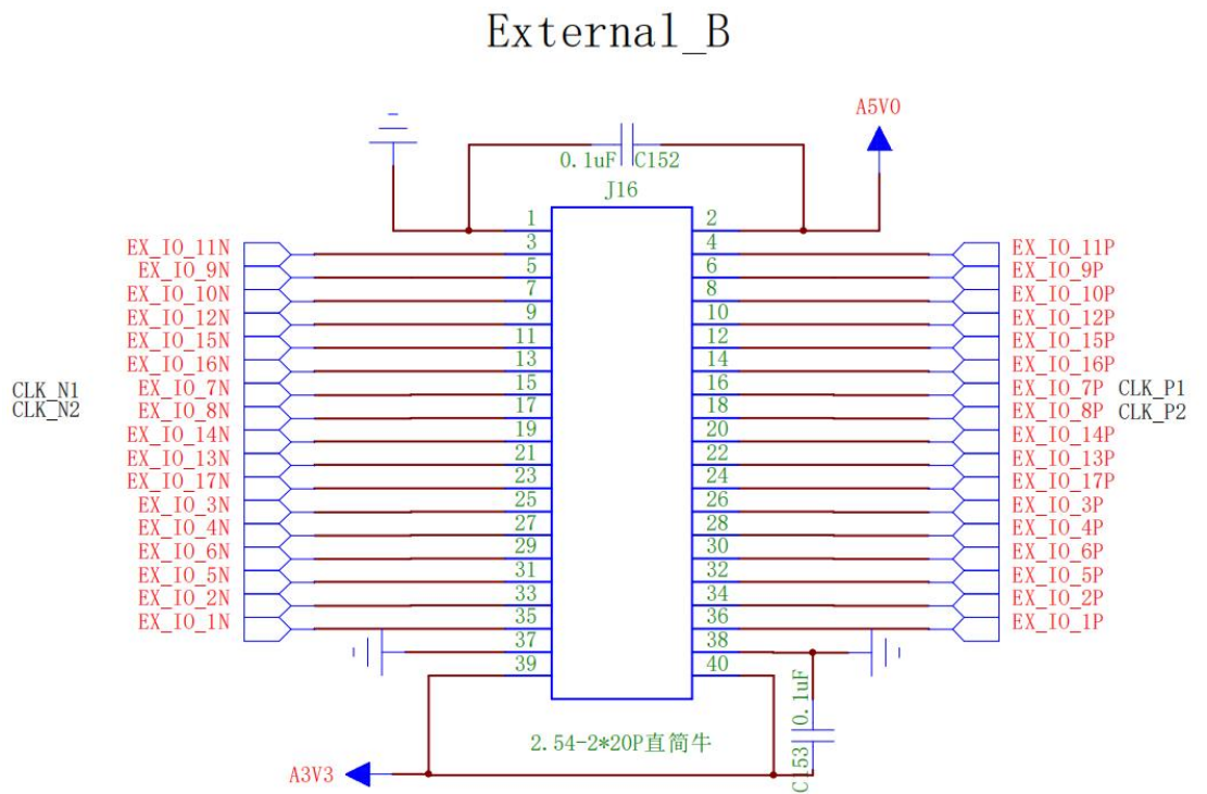
图 3-8 40pin 扩展 IO 原理图
