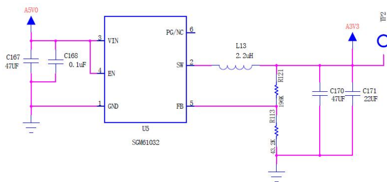
图 3-10 5V 转 3.3V 原理图
