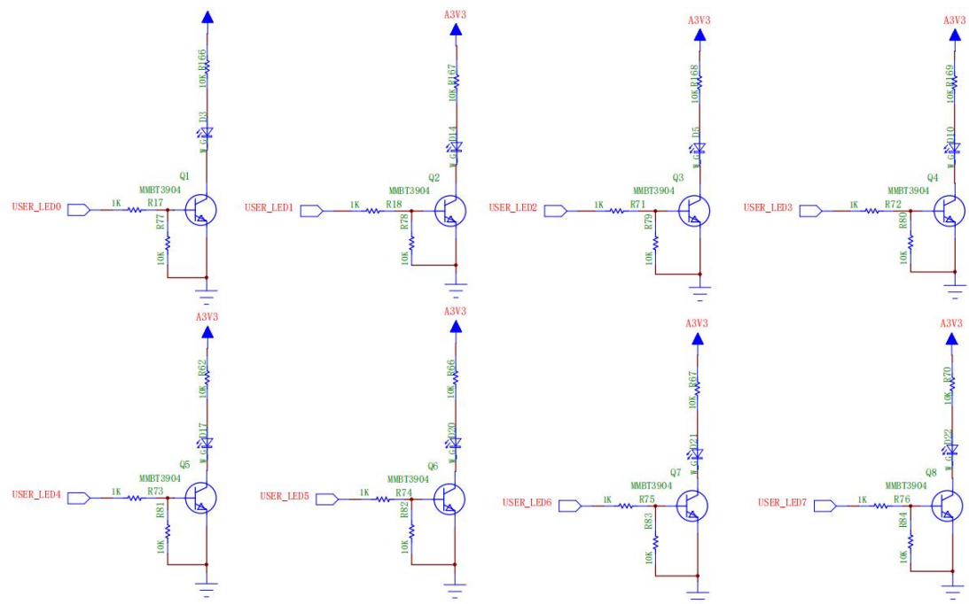
图 3-7 LED 灯电路原理图
