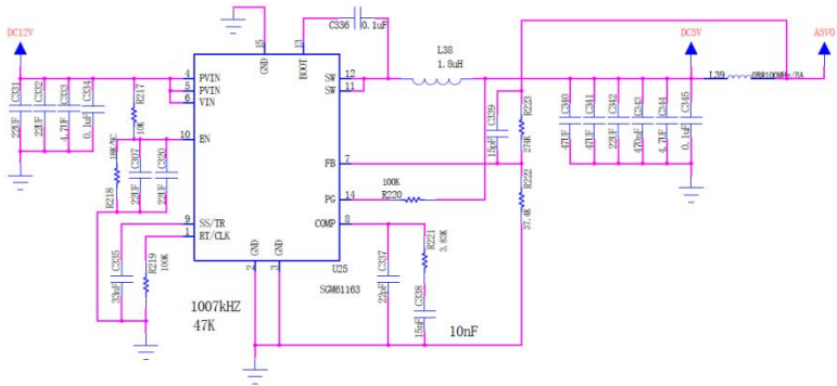
图 3-9 12V 转 5V 原理图
