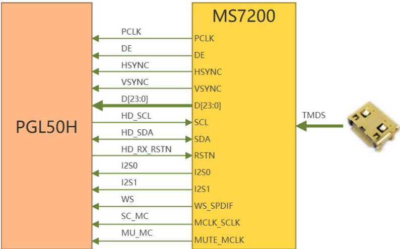
图 3-4 HDMI Receiver 连接示意图
