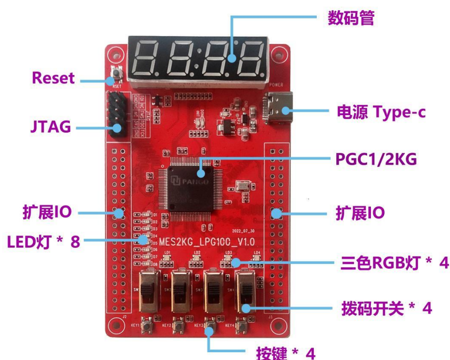
图 1.1 MES1/2KG 开发板
